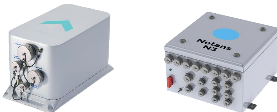
Système de navigation composé d'un gyrocompas Octans et d'un Netans NDDS (Navigation Data Distribution System)
