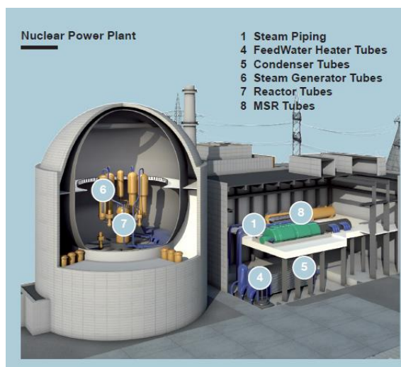
Les tubes de Vallourec dans une centrale nucléaire
