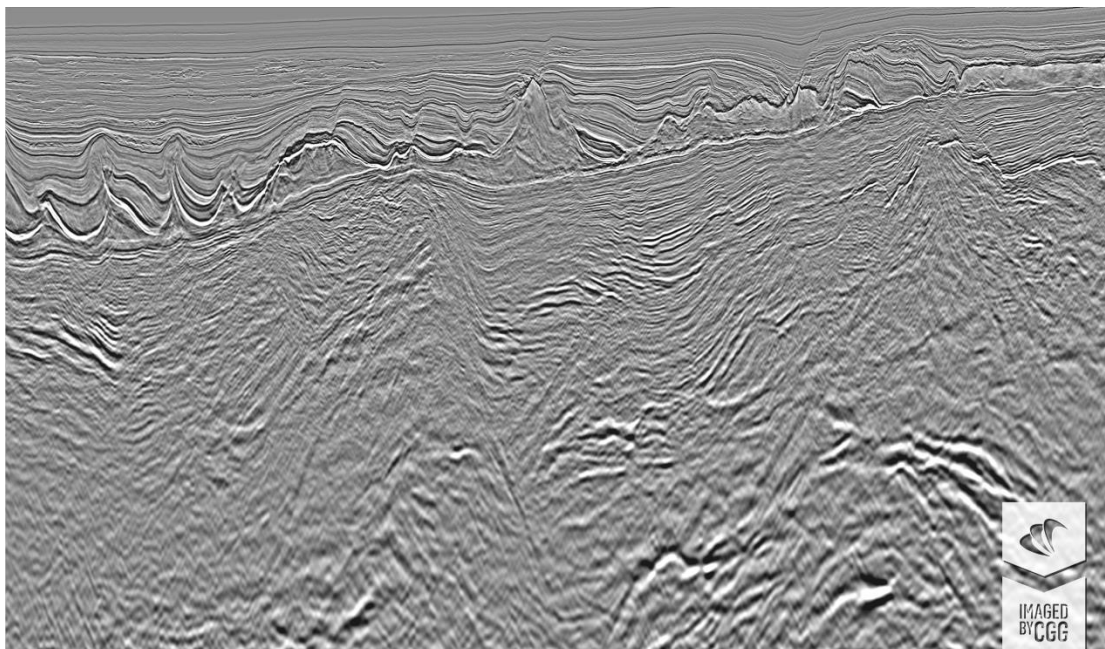
Coupe sismique Kirchhoff PreSDM finale montrant un large fossé pré-salifère constitué de sédiments visibles jusqu'à 12 km de profondeur ainsi qu'au niveau de la base du sel des structures géologiques à fort potentiel (source : CGG Multi-Client & New Ventures).
