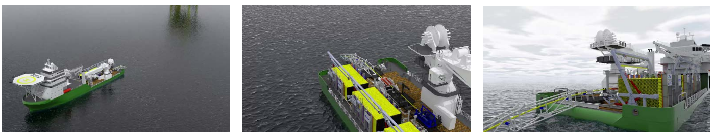
Vues 3D réalisées par Cortez du Bourbon Evolution 800 avec le spread de pose de pipeline.
