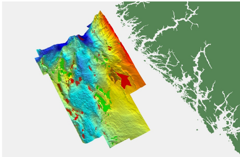
La Discordance basale du Crétacé interprétée à partir de l'étude multi-clients 'Northern Viking Graben' de CGG.
